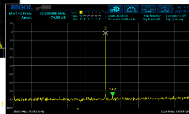
-70 dBc SFDR
